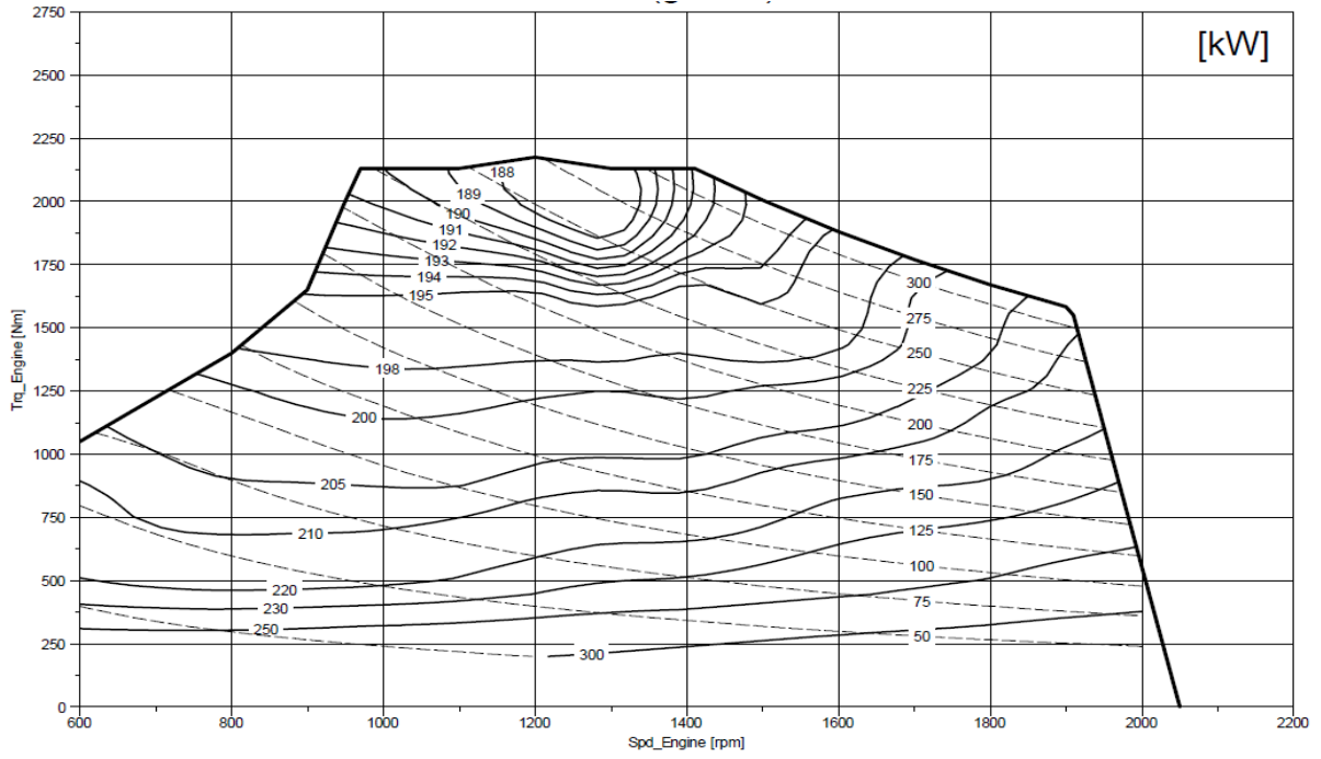
BSFC [g/kWh]
